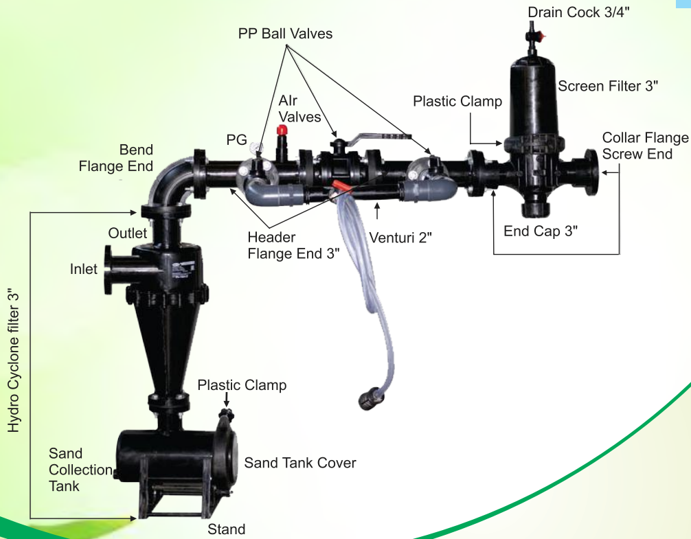
HydroCyclone (2", 2.5", 3")
